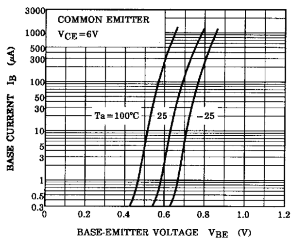
Fig. 8.6 I_B - V_{BE}
