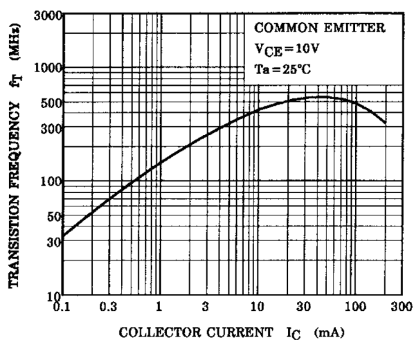
Fig. 8.5 f_T - I_C
