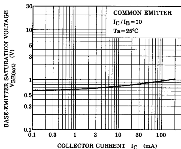
Fig. 8.4 V_{BE(sat)} - I_C
