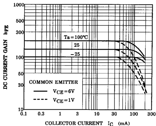
Fig. 8.2 h_{FE} - I_C
