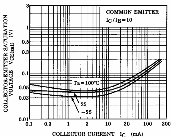
Fig. 8.3 V_{CE(sat)} - I_C
